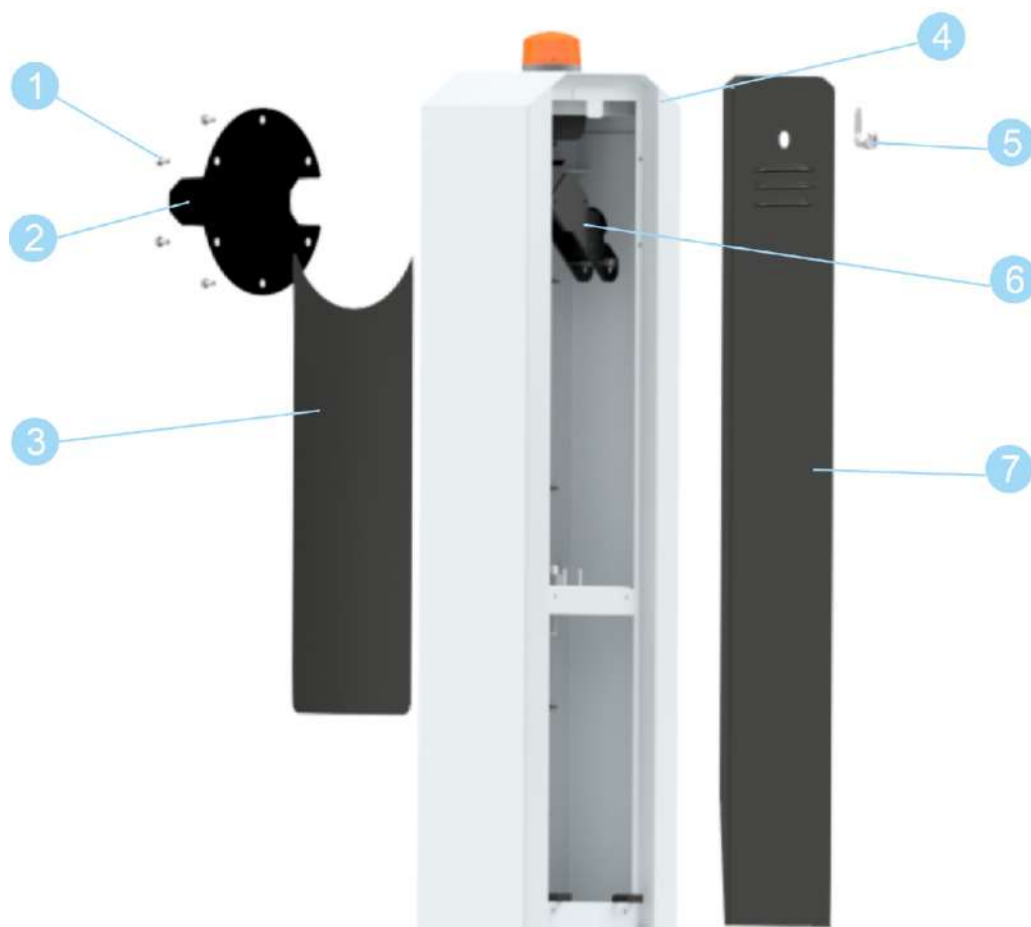
Рисунок 6.1.1 Внешний вид и состав корпуса шлагбаума
